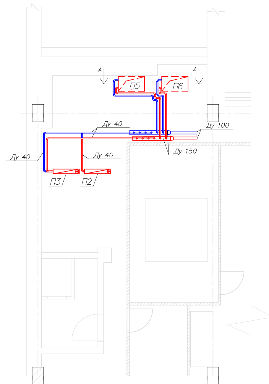
План 2-го этажа
