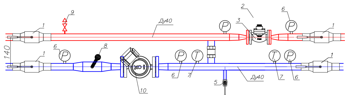
Узлы обвязки П1-П6
